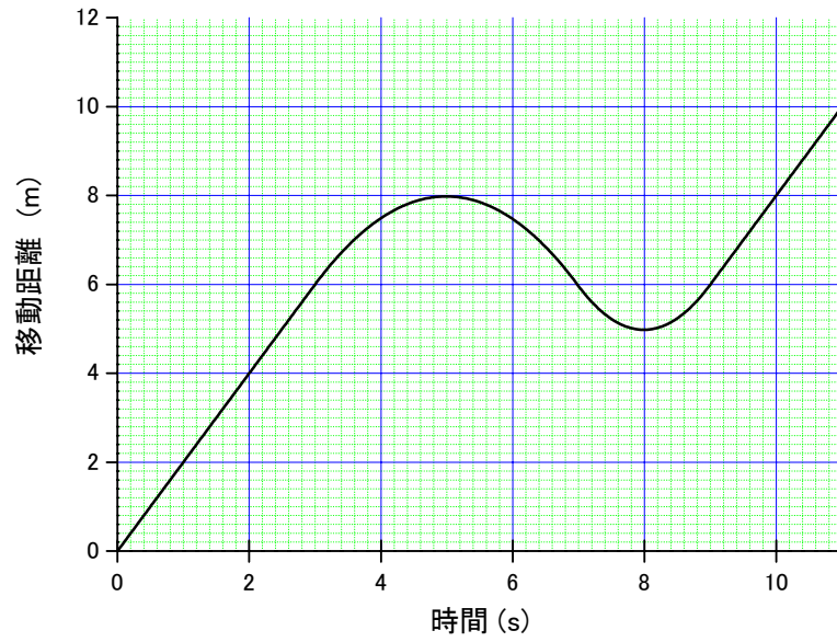
運動する物体の位置の時間依存性
