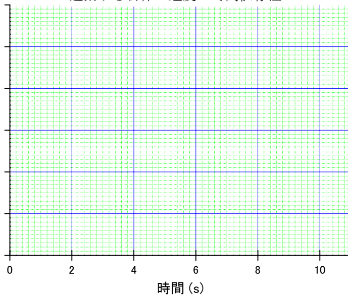
運動する物体の速度の時間依存性
